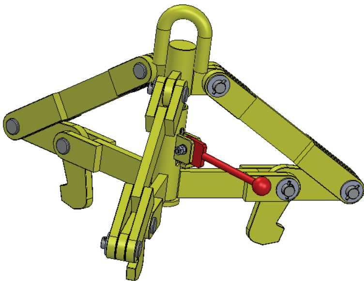
PINZA DI SOLLEVAMENTO MATASSE / FOIL ROLLS LIFTING CLAMP PORTATA / CAPACITY 2.500 Kg
