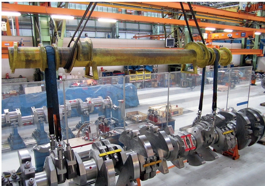
BILANCINO SOLLEVAMENTO ALBERI / CAMSHAFT LIFTING BEAM PORTATA / CAPACITY 50.000 Kg
