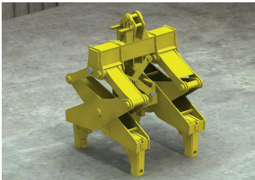
PINZA DI SOLLEVAMENTO BRAMME / SLABS TONG PORTATA / CAPACITY 10.000 Kg
