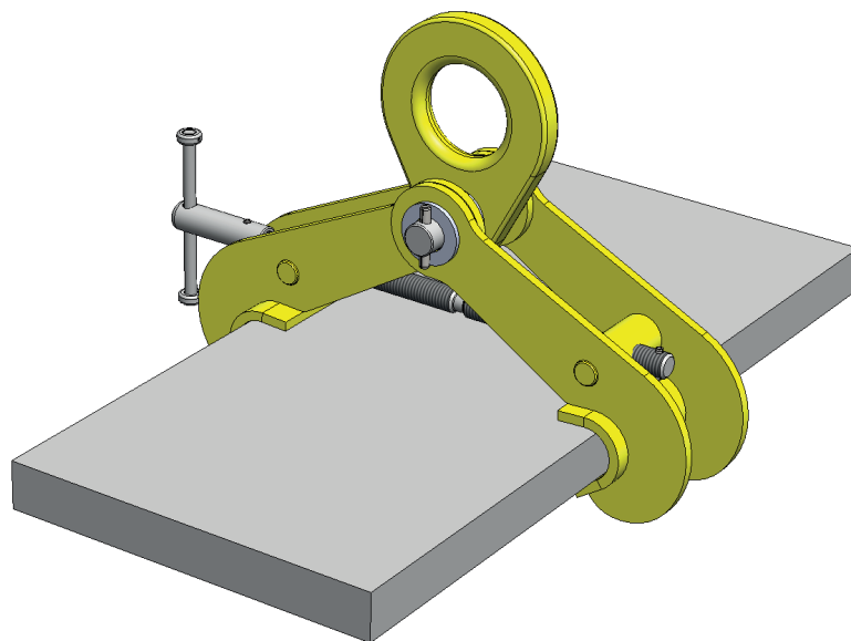
PINZA DI SOLLEVAMENTO TRAVI / LIFTING CLAMP PORTATA / CAPACITY 5.000 Kg
